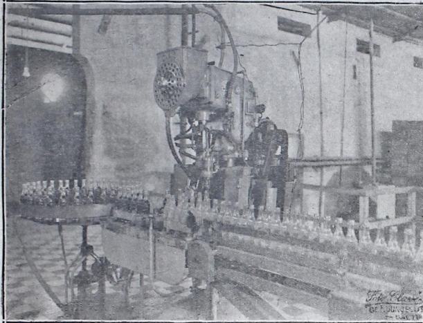
Modernísima máquina automática llenadora y tapadora de envases de bebidas sin alcohol
