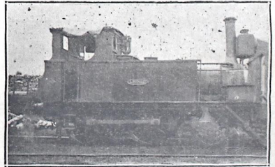
Máquina "Criollo" construida totalmente en los talleres del F. C. N. O. en el año 1895. Actualmente es la destinada a correr trenes expresos y ha llegado a andar a una velocidad aproximada a cien kilómetros por hora.
